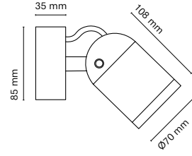
24810- Far Wall 70
