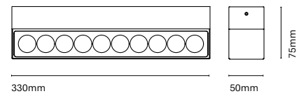
24452- Vlok Wall
