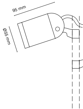
24812- Far Modular 55
