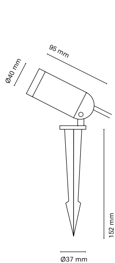
24805- Far Spike 40
