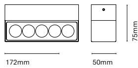
24446- Vlok Wall
