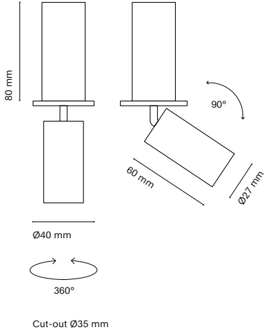
06814- Telos 40
